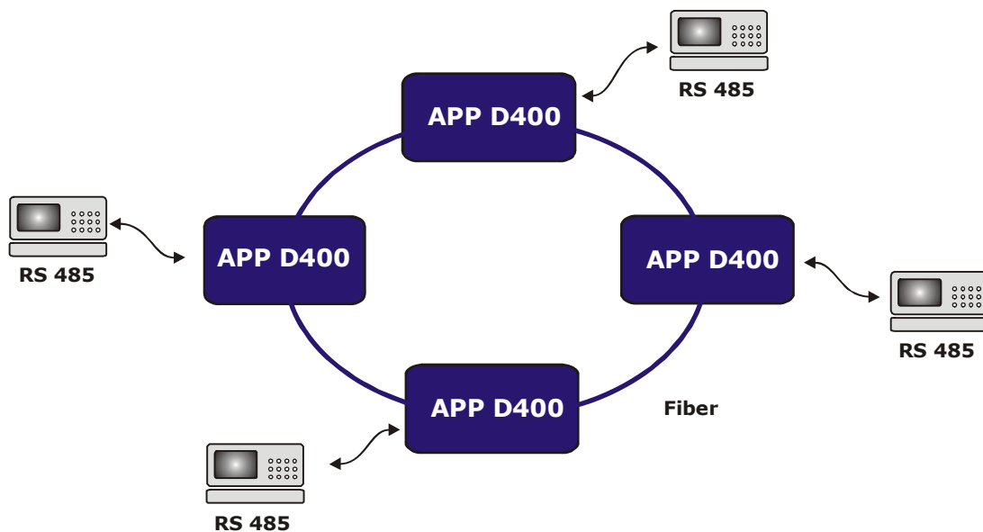
Rysunek 4. Przykładowa instalacja APP D400 w topologii pierścienia z redundancją połączenia optycznego
