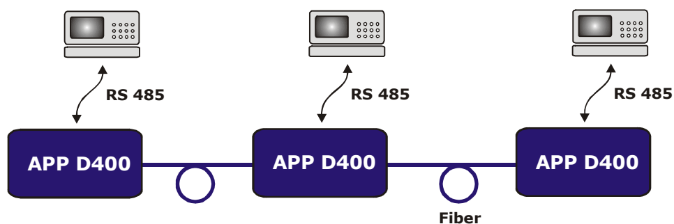
Rysunek 3. Przykładowa instalacja APP D400 w topologii magistrali
